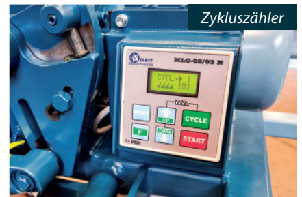
Abziehvorrückung Schleifscheibe
